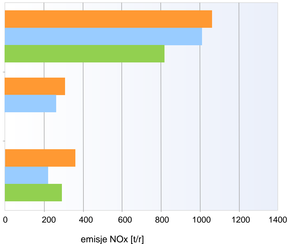
ogrzewanie budynków
